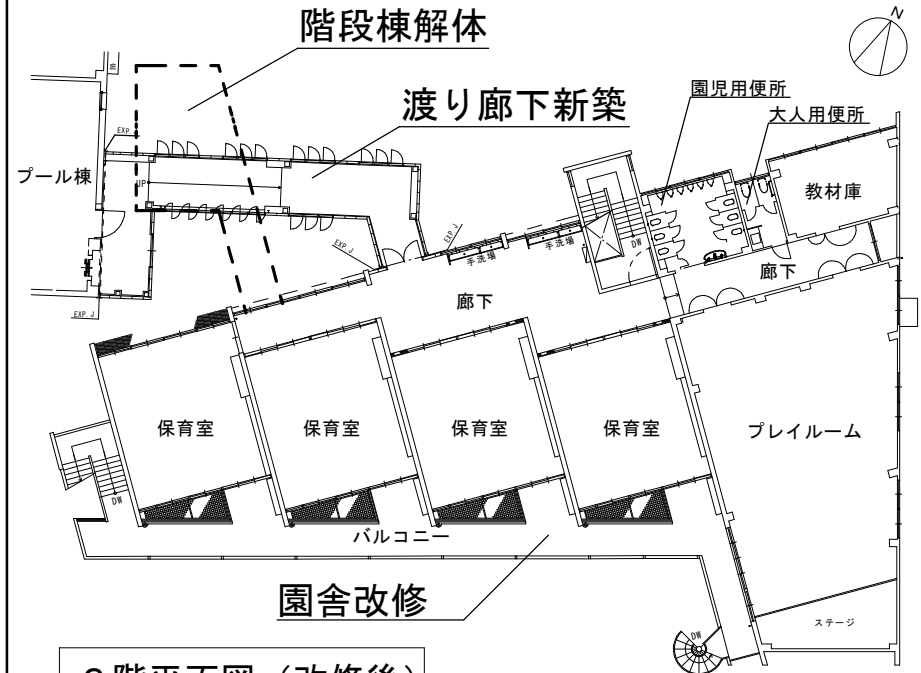
2階平面図 (改修後)
