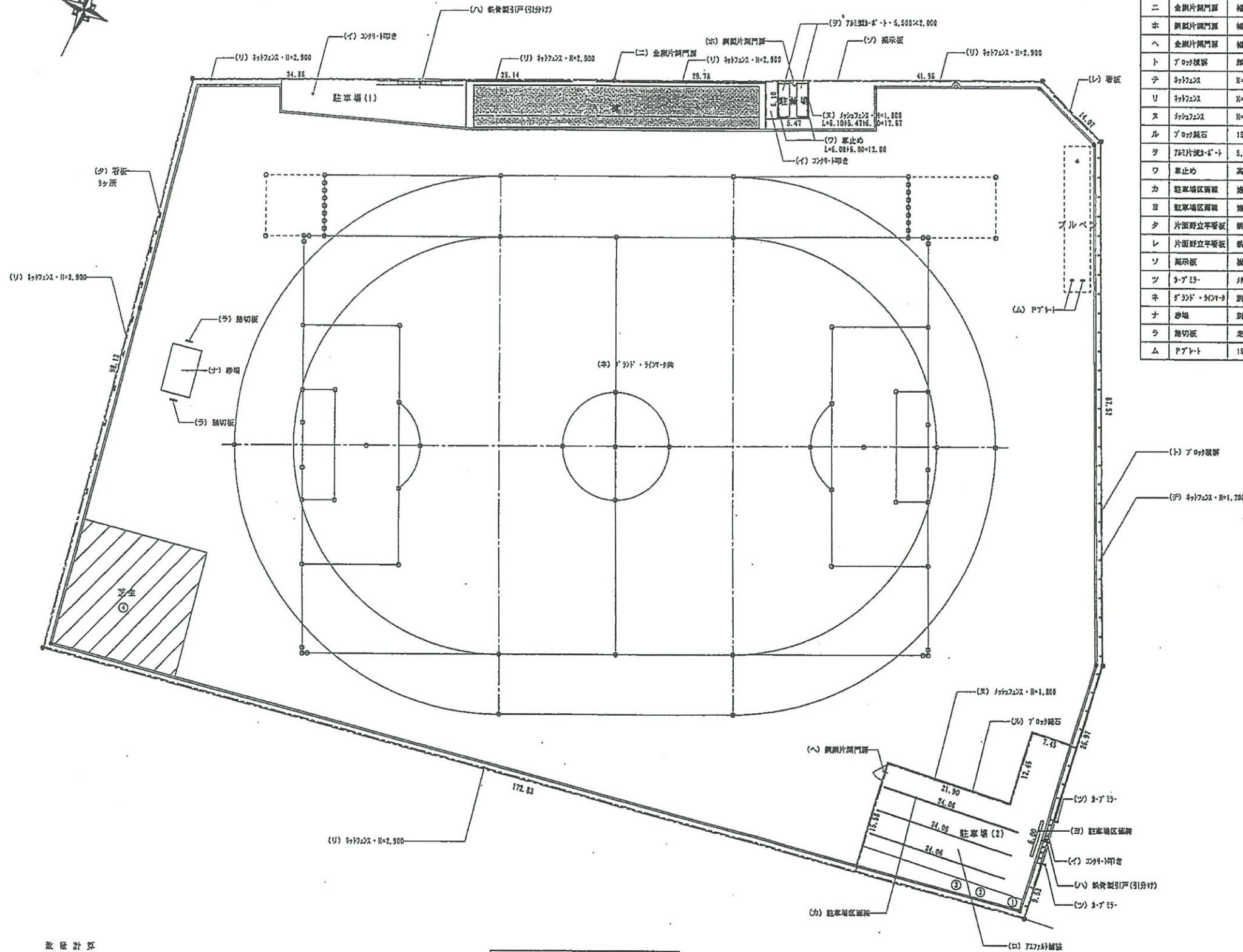
配置図 1/500
