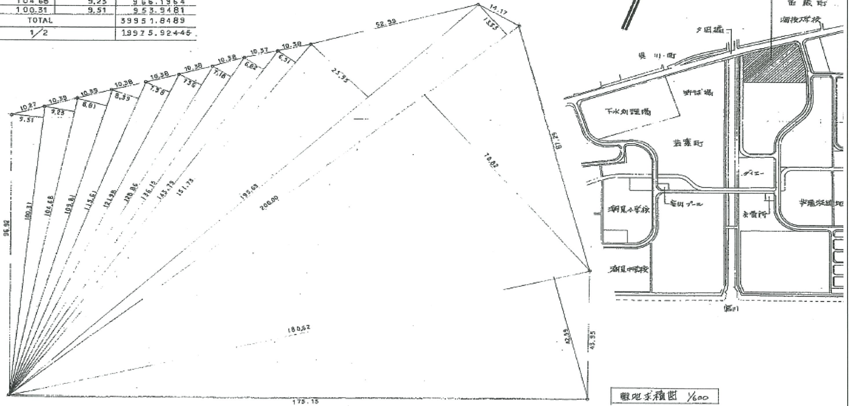
別添資料 1-2 敷地求積図
