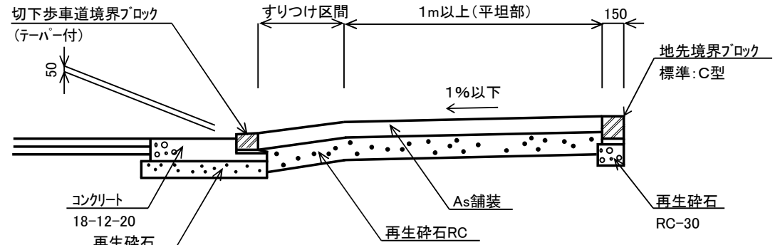
舗装断面図 ※As舗装の場合
