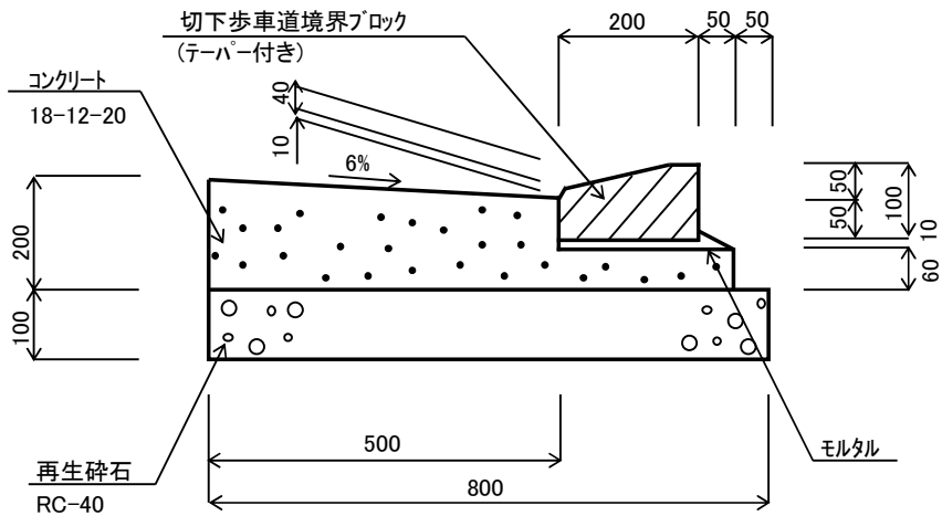
街渠構造図（切り下げ部）
