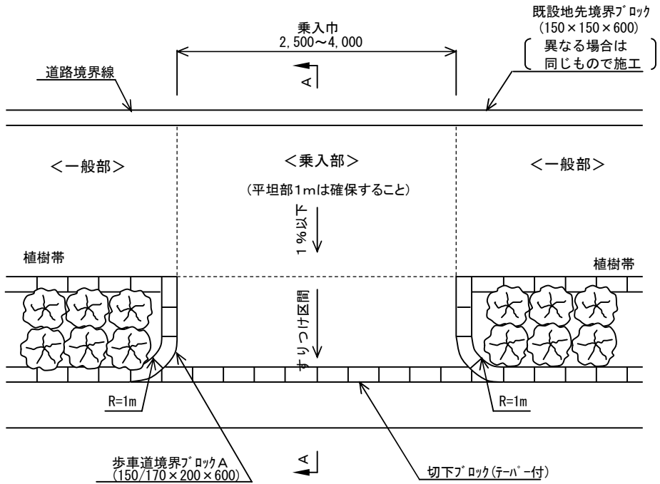
平面图
