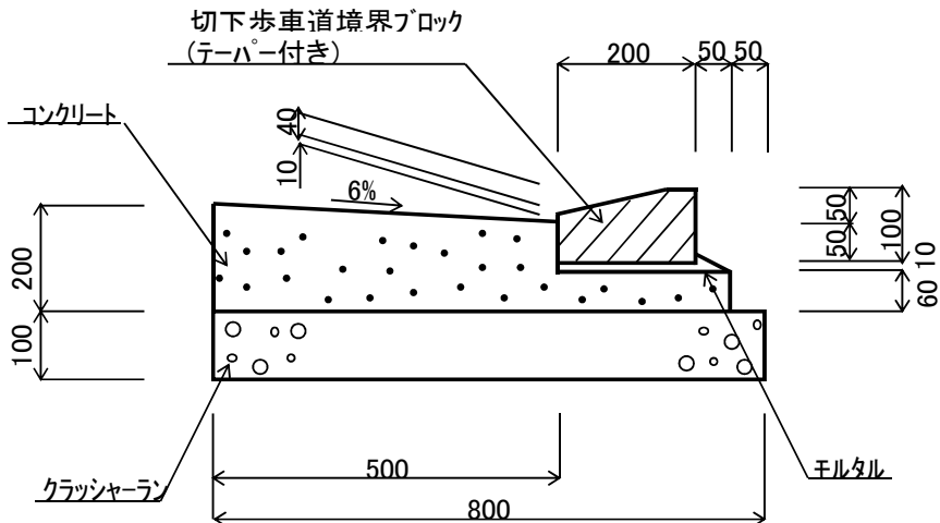
切下歩車道境界ブロック部構造図
