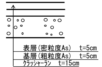
歩道（乗入れ部）4t車以上
