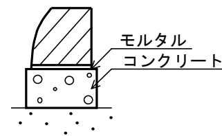
歩車道境界ブロックA構造図
