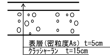
歩道（乗入れ部）4t車未満
