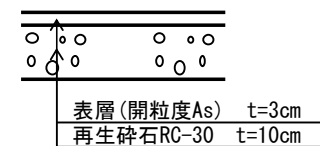
歩道（一般部）
