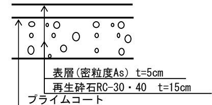
歩道（乗入れ部）4 t以上
