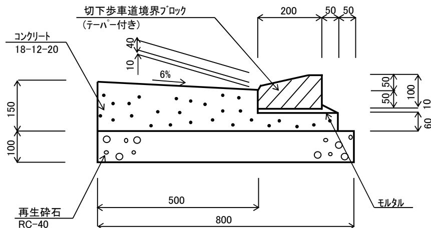
街渠構造図（切り下げ部）
