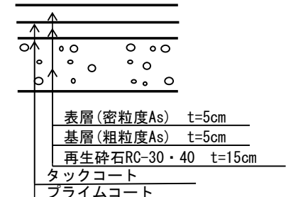
歩道（乗入れ部）4 t以上
