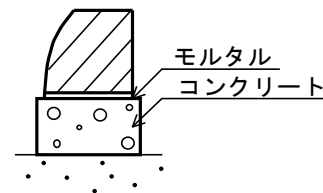
歩車道境界ブロックA構造図
