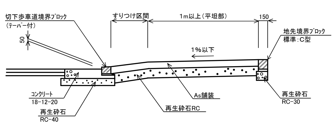
舗装断面図 ※As舗装の場合
