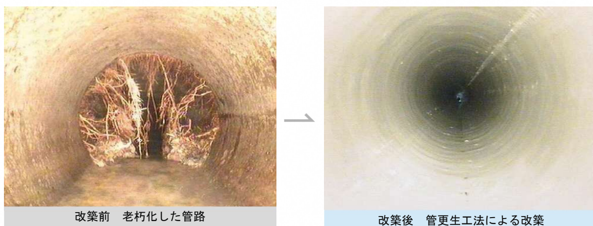
写真 7 管路の改築状況
