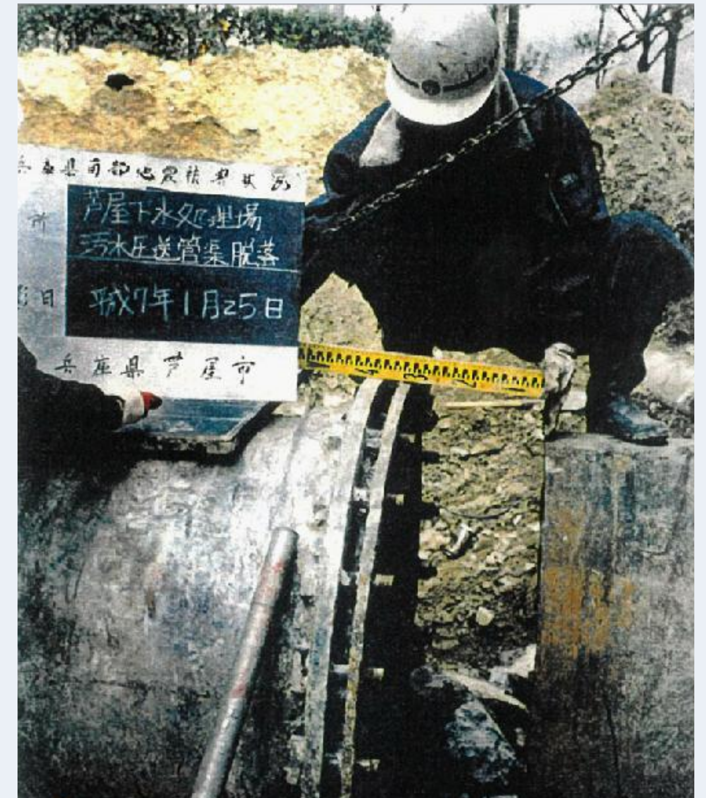
汚水管路の脱落
