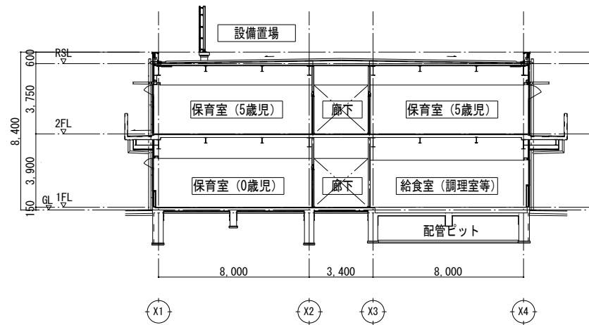
A断面図
