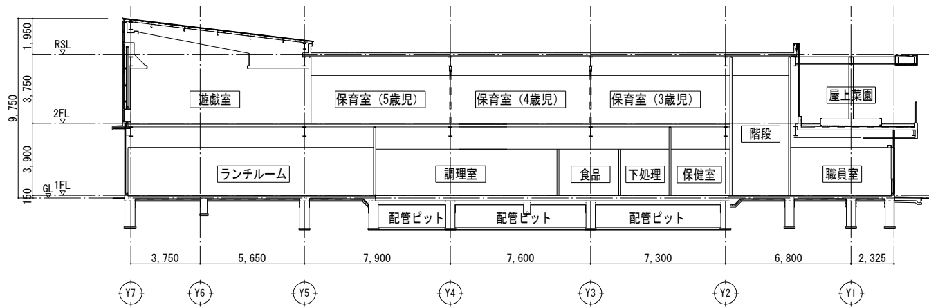
B断面図
