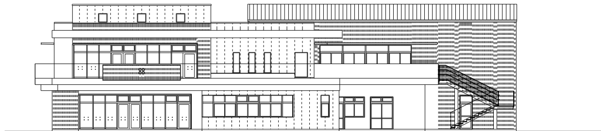
南立面図
