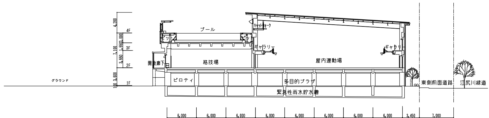
C断面図
