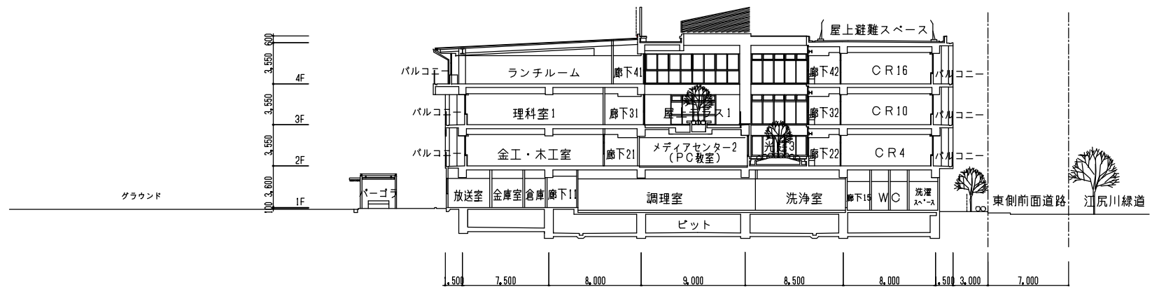
D断面図
