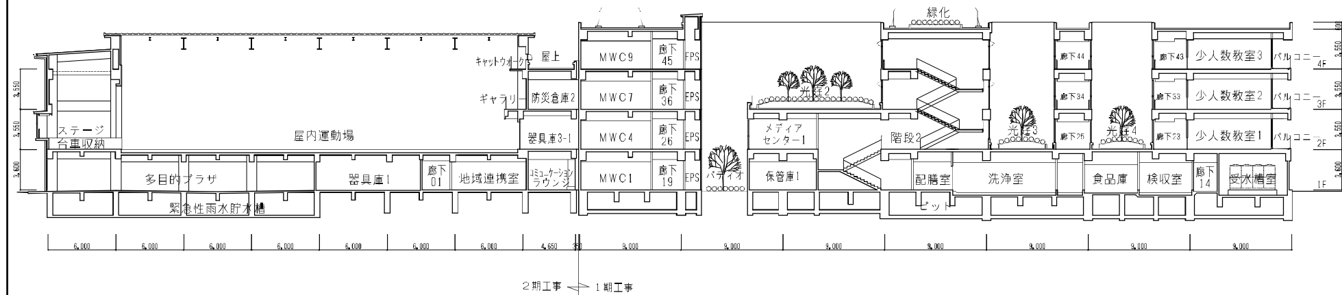
B断面図
