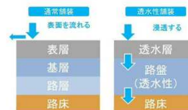
通常舗装と透水性舗装の違い
