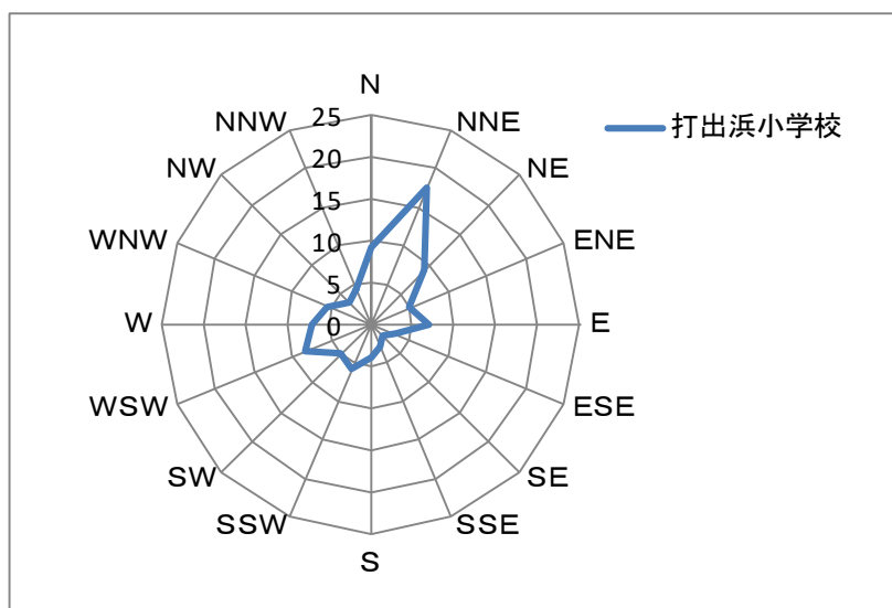
図 2 - 6 風配図 (単位 : %)
