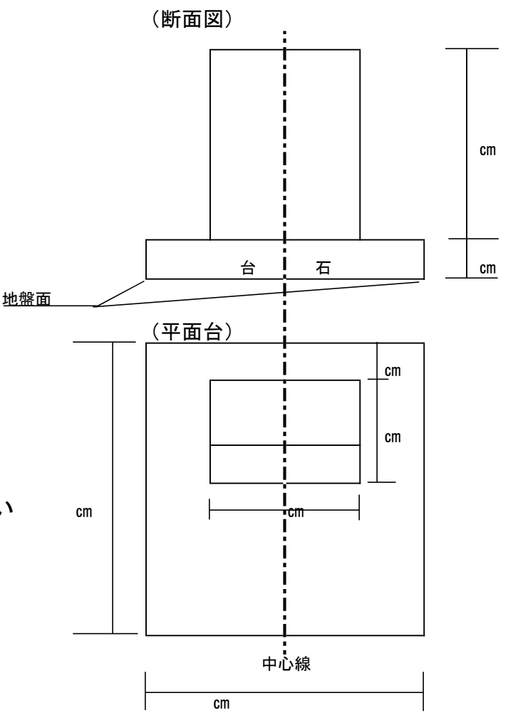
芝生霊園設計図
