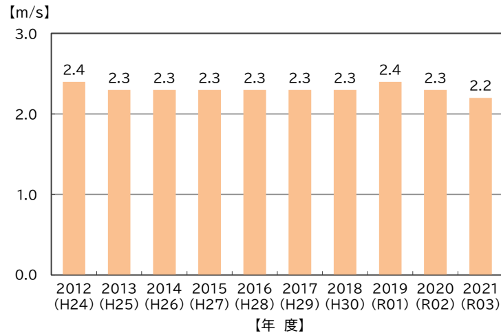
年間平均風速の推移 (資料：芦屋市統計書)
