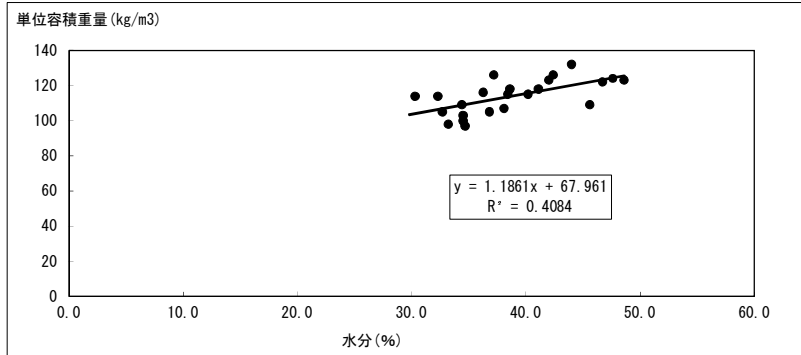
図 7-1-5 単位容積重量と水分の相関
