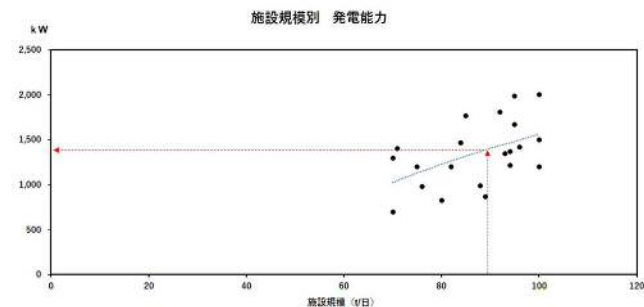
図－１ 施設規模別の発電事例（参考）（環境省 HP より作成）
