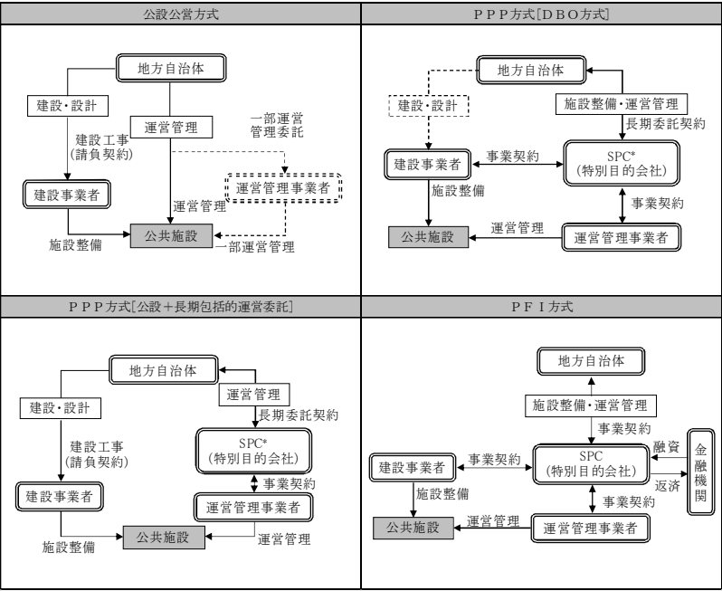
図 16-1 事業方式別の概略フロー
