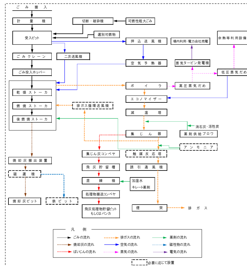
図－2 処理フロー図（想定）
