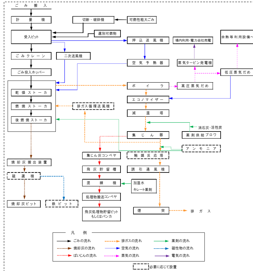
図 13-2 処理フロー図 (想定)
