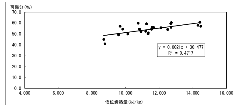
図 7-1-4 低位発熱量と可燃分の相関
