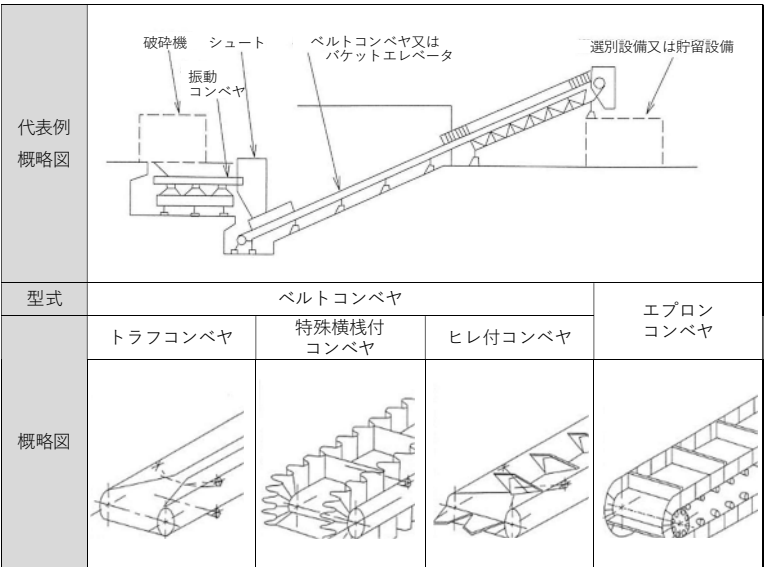
図 8-2-2 搬送設備の代表例及び概略図
