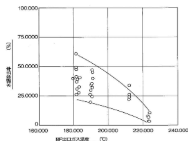
図－１ ろ過式集じん器（バグフィルタ）出口温度と水銀除去率
