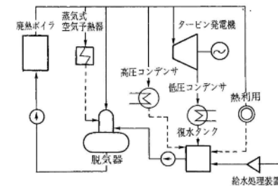
復水タービン（例）※
