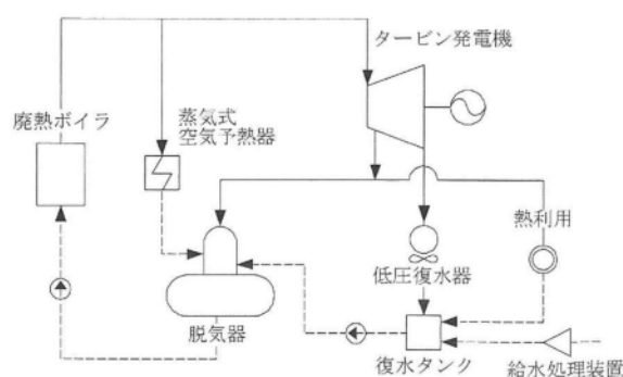
全量発電の場合のフローシート例
