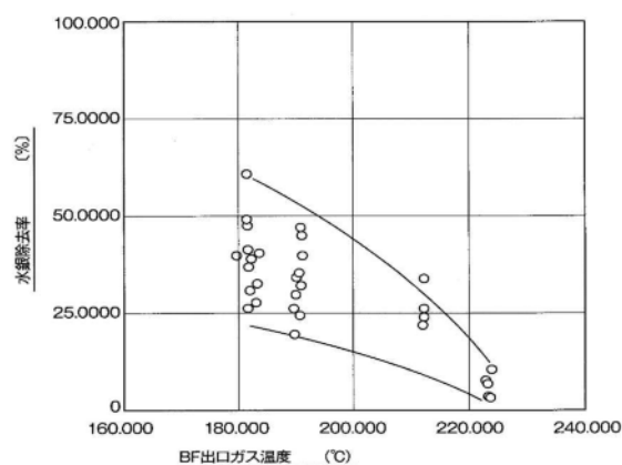
図ー１ ろ過式集じん器（バグフィルタ）出口温度と水銀除去率
