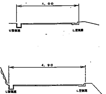
標準断面図 S=1:100
