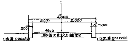
A-A 断面図 S.1:100
