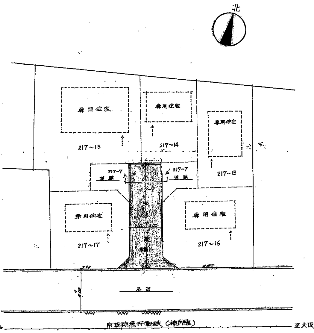
配置図 S.1:200
