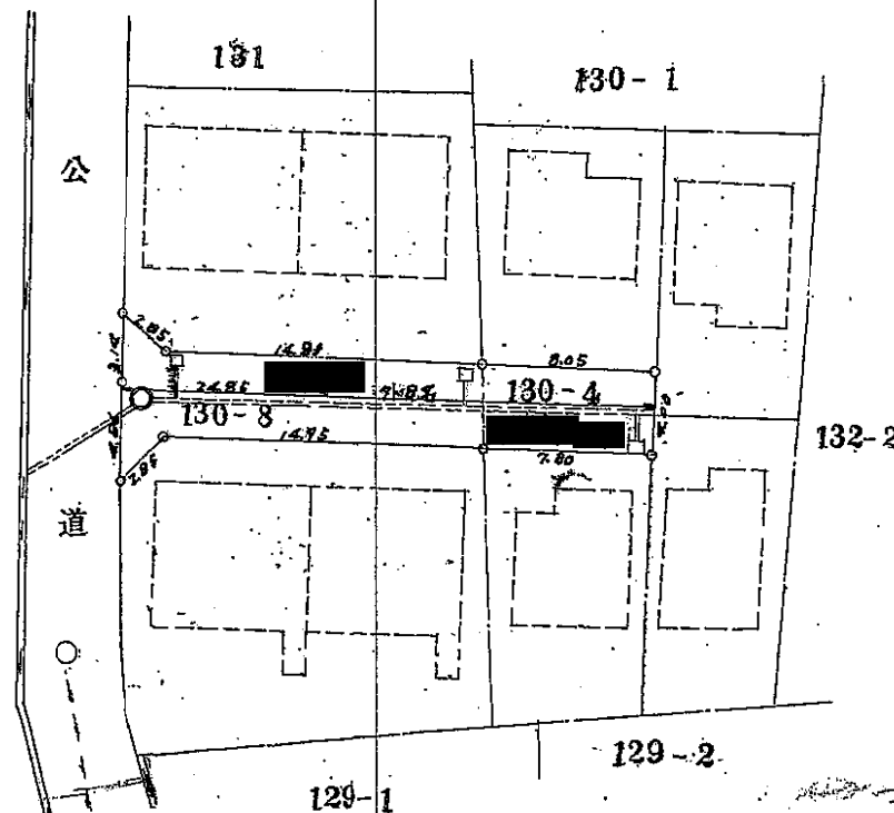
平面図 S=1/500
