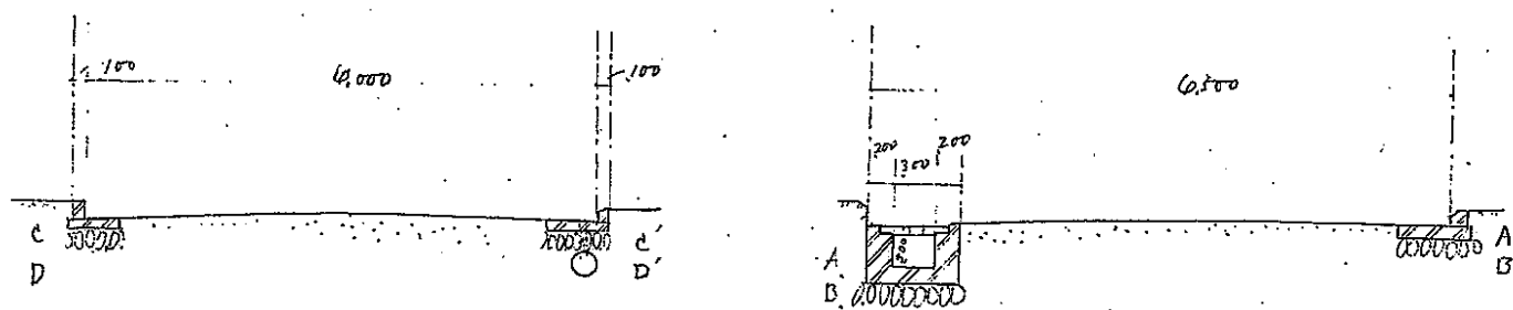
標準断面図 1:50
