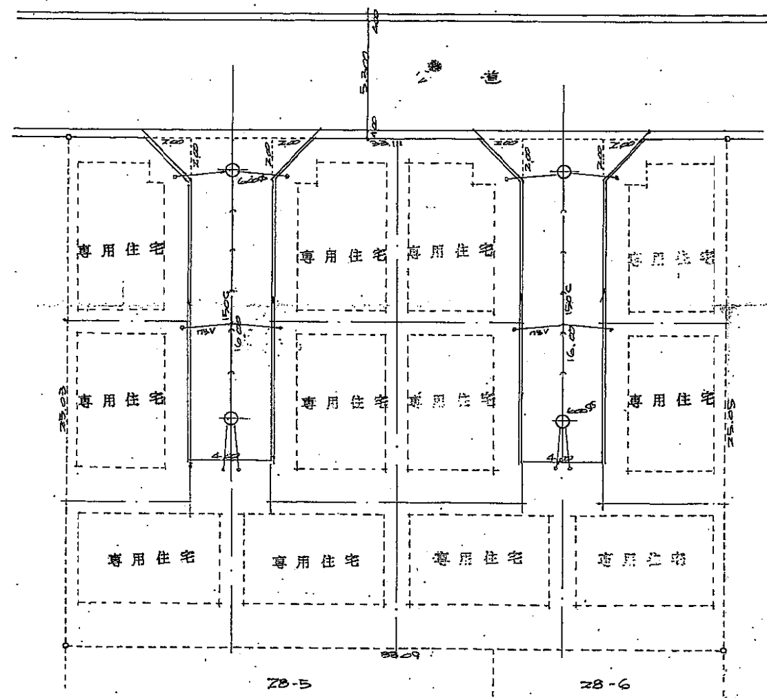
平面図 S:200
