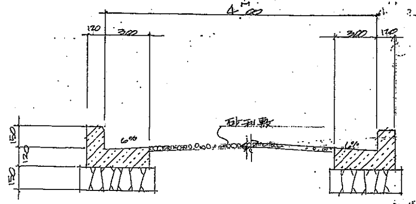
断面図 S:20
