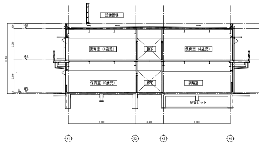
A断面図
