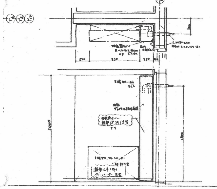
(參考圖) 本圖施工範圍在左表以上。 1:30
