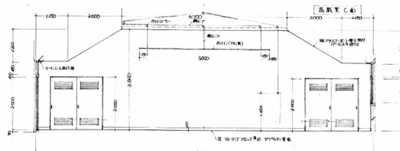
遊戯室 D面
