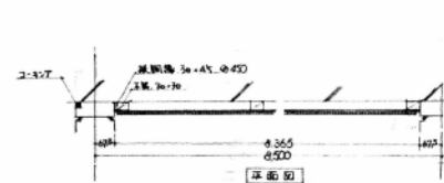
2階 候鳥室平面詳細図 1/50
