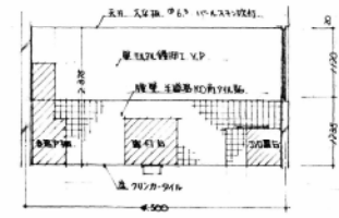
飲食室 D 面
