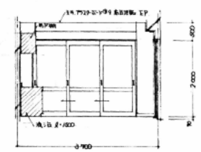
接客室 C 面
