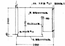
接客室 J 面
