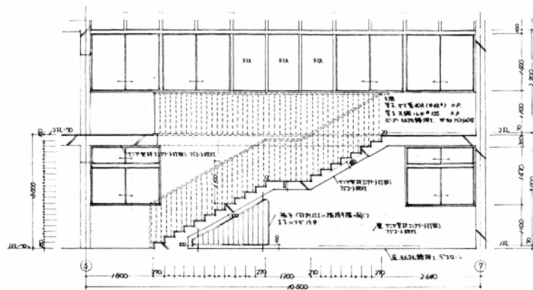
1階階段詳細図 1/30
