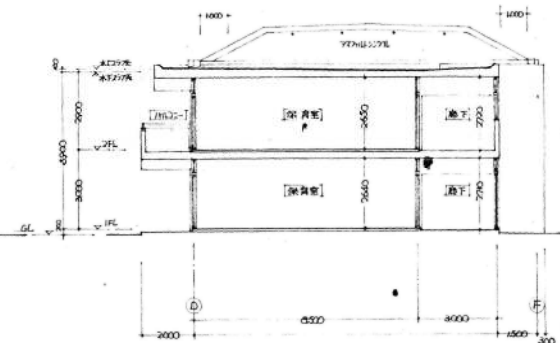
7~8 断面図
