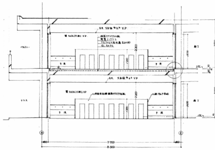
児童遊具用床 A面
