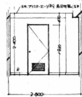
接客室 H 面
