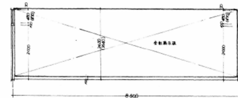
2階 候鳥室平面詳細図 1/50
