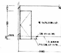
用務員室C断面
