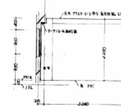
用務員室A断面
