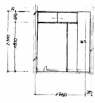
用務員室E断面
