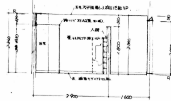
用務員室F断面
