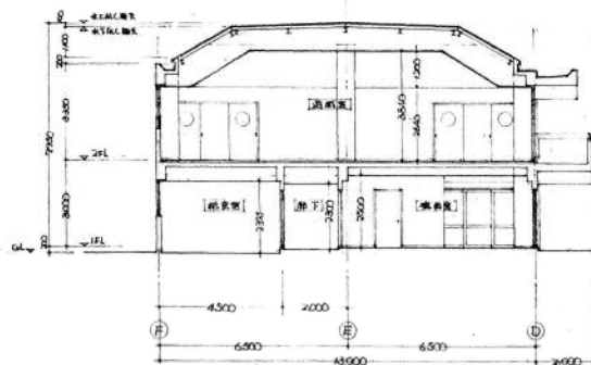
2~3 断面図
