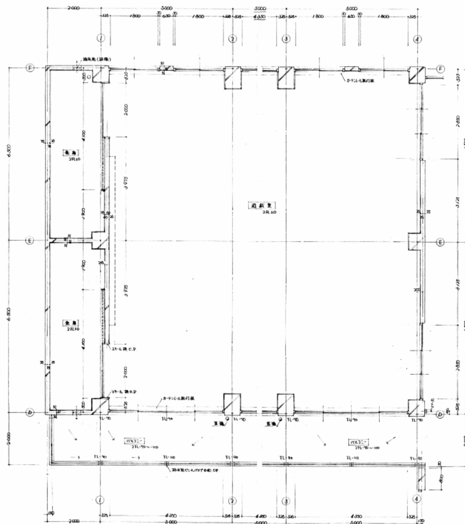
遊戯室入り平面詳細図 1:1/30
