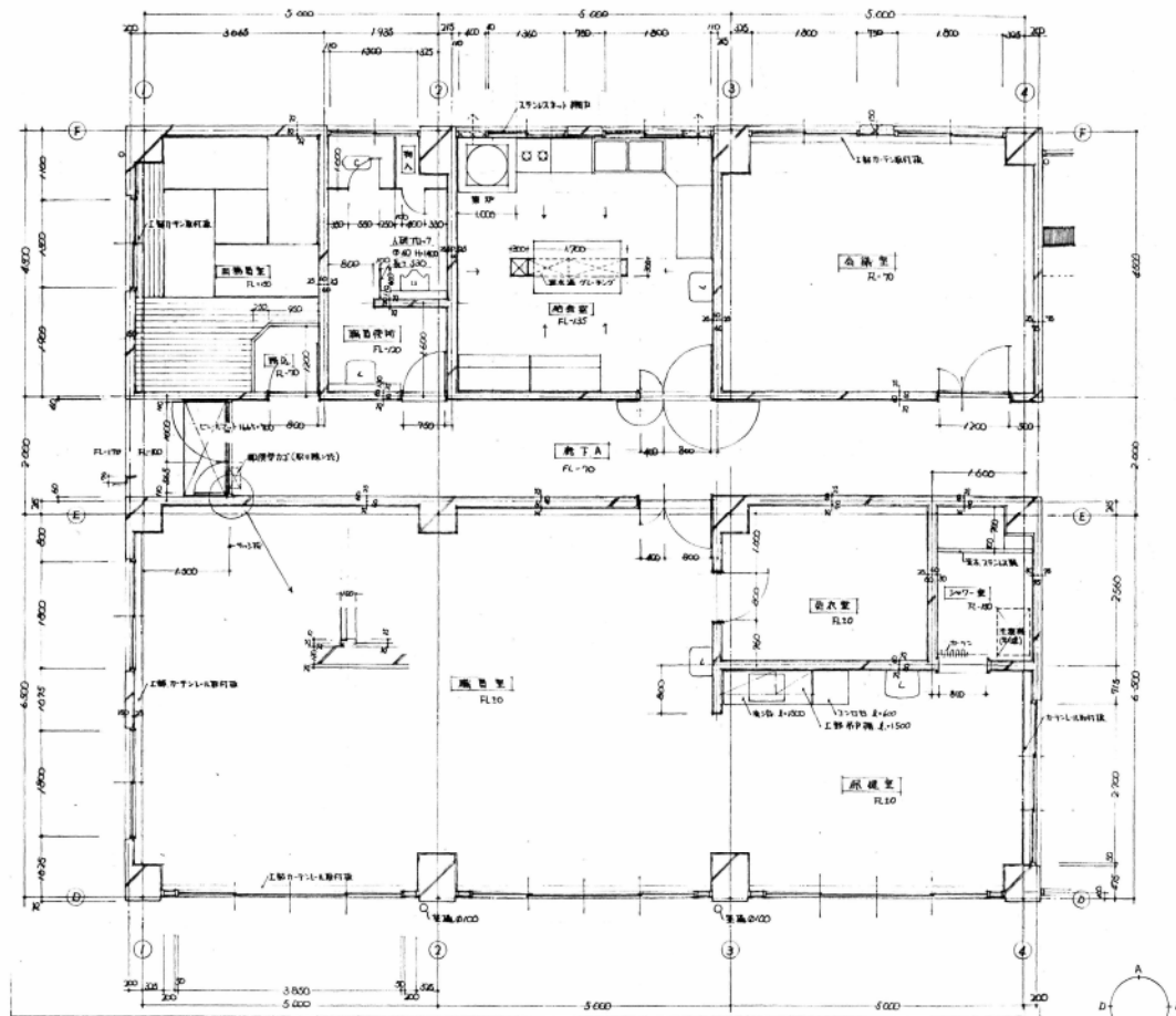
食堂廻り平面詳細図
