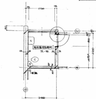
部分詳細図 1/30
