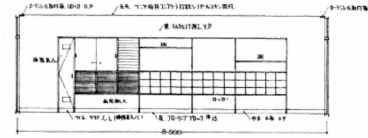
2階 候鳥室平面詳細図 1/50
