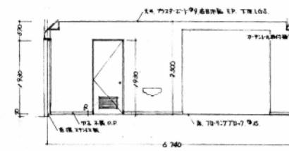
接客室 B 面
