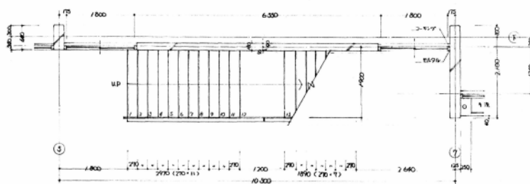
2階平面詳細図 1/30
