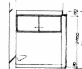
特別児童遊具用床 A面 1/30
