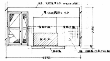
飲食室 C 面
