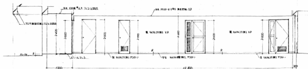
廊下A断面
