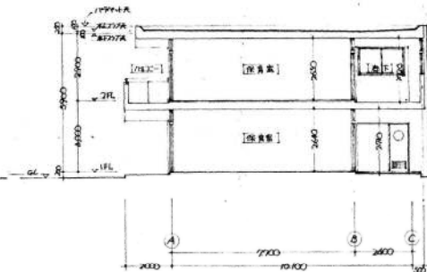
11~12 断面図
