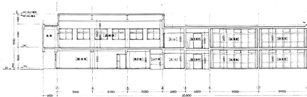
D~E 断面図
