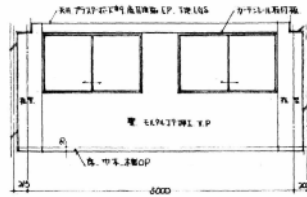
会議室 A 面
