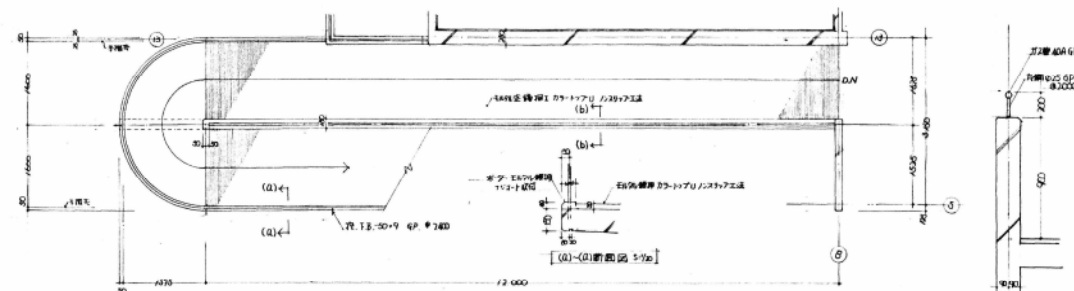
2階平面詳細図 1/30
