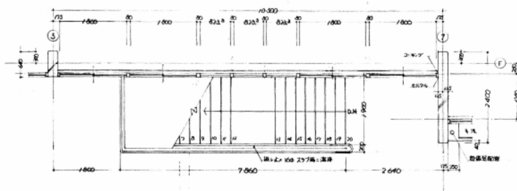
2階平面詳細図 1/30
