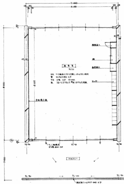
2階 候鳥室平面詳細図 1/50
