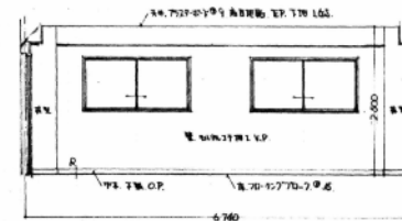
接客室 E 面
