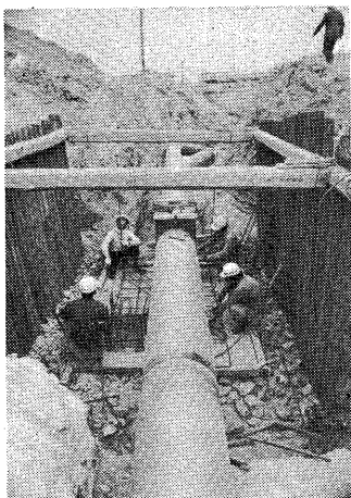
布設工事の現場
