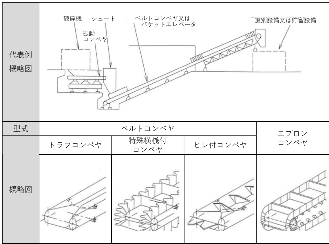
出典)「ごみ処理施設整備の計画・設計要領 2017 改訂版 P.638」公益社団法人 全国都市清掃会議 図 8-2-2 搬送設備の代表例及び概略図
