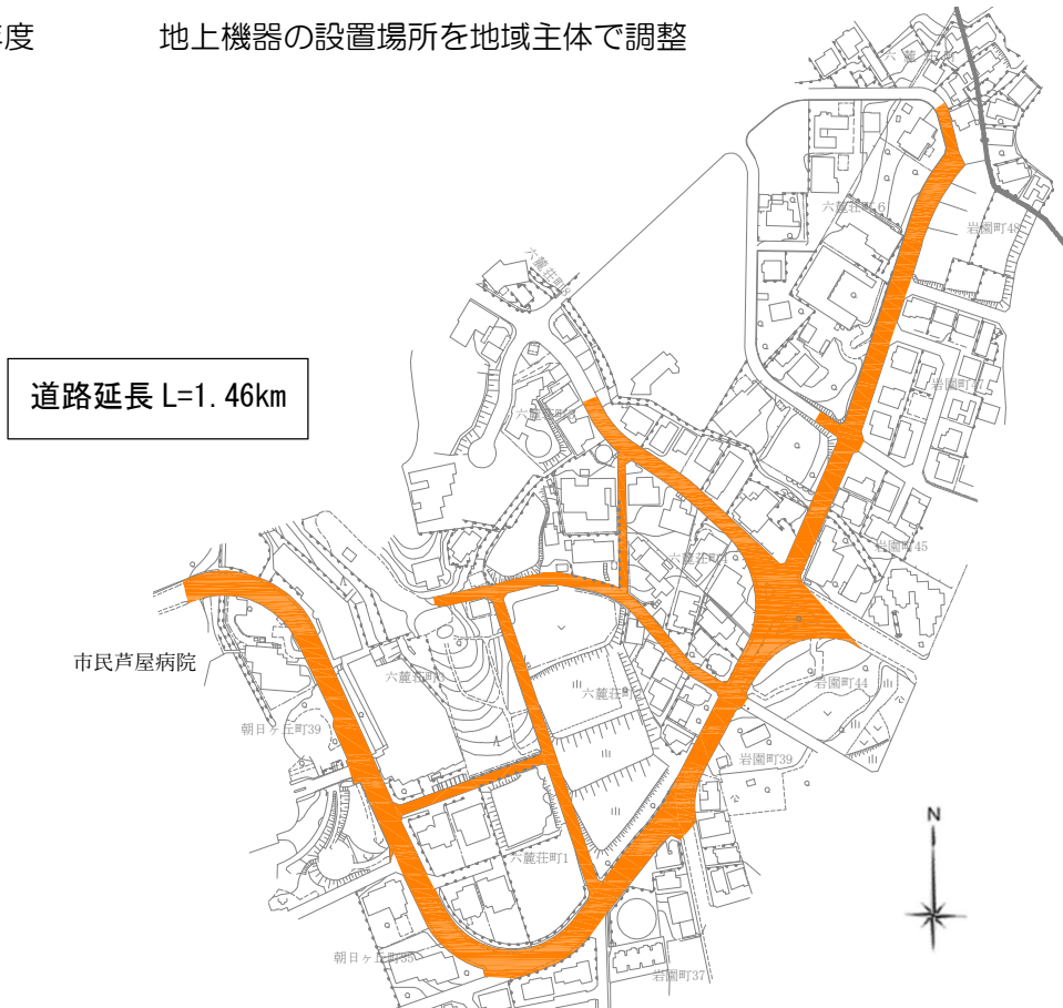
図 六麓荘地区における無電柱化計画路線
