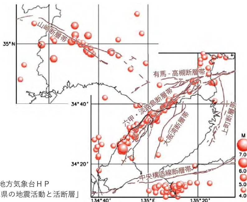
図 - 活断層と地震活動（1919年以降の地震を表示）
